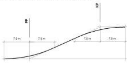
Слика 12. Проширување со заоблување
