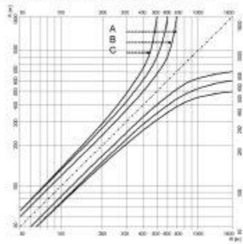
Слика 29. Односи на редоследот на радиусите на лациите
