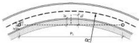
Слика 25. Шематски приказ на полето на хоризонталната прегледност.
