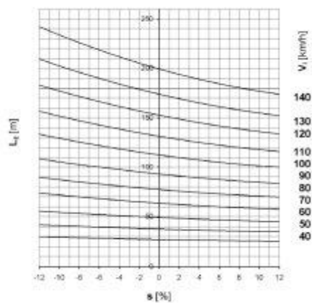
Слика 22. Прегледност за застанување на коловоз со одвојување на групите А.
